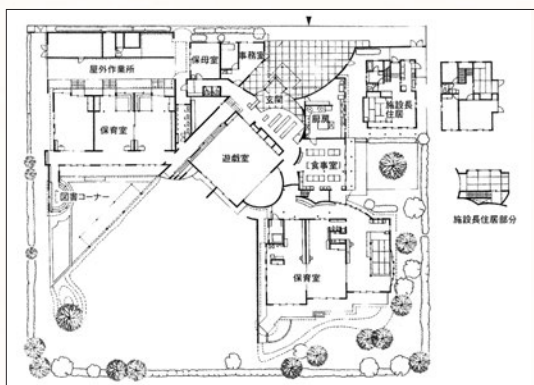
保育園るんびいに(小川信子設計)
