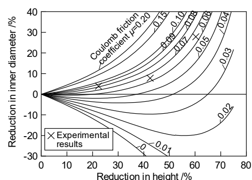
図1 摩擦係数の同定
