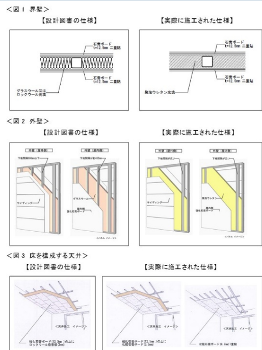
図：建築基準法仕様不適合事例：国土交通省HP
