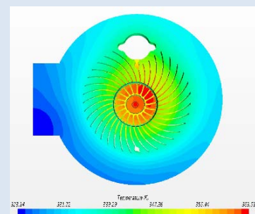
数値シミュレーションによる温度分布の様子
