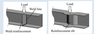
従来溶接構造 開発一体構造 塑性と加工 45巻524号 pp. 737-741
